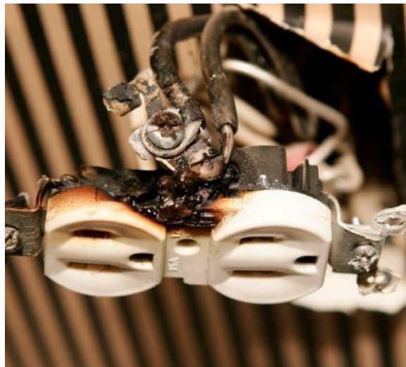
Photo F1 – Failure of aluminum wiring terminations
